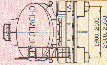
А Вариант исполнения 3
