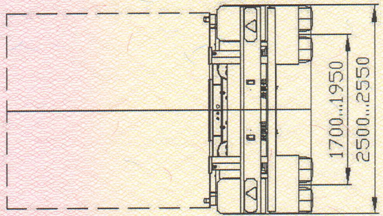
А Вариант исполнения 2
