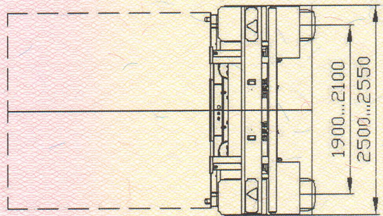
А Вариант исполнения 1
