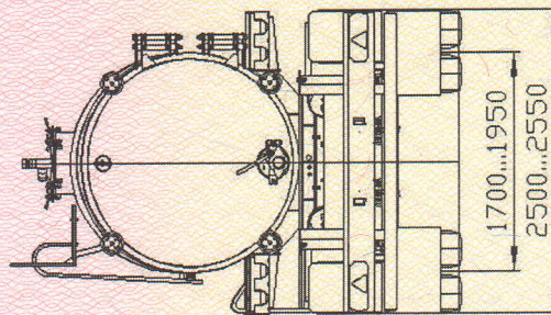
А Вариант исполнения 16
